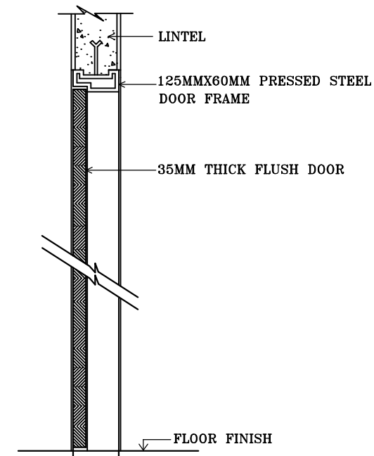
SECTION YY N.T.S.
