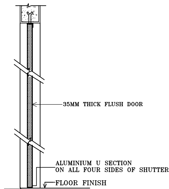
SECTION AT Y'-Y' N.T.S.
