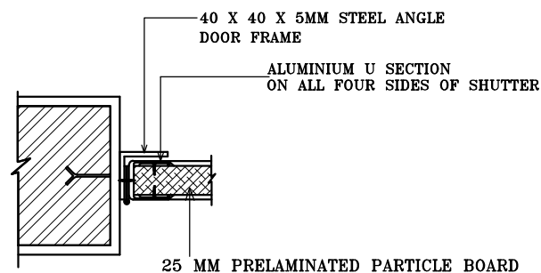
DETAIL AT A N.T.S.
