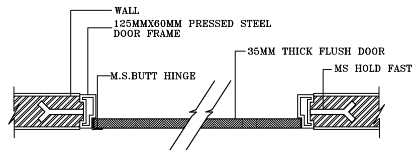
SECTION XX N.T.S.
